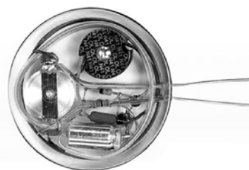
Primer marcapasos implantable realizado en 1958.
