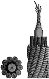
Estructura de un cable submarino.
